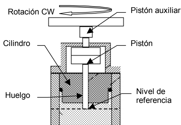
Figura 1 ensamble pistón cilindro reentrante [6]
