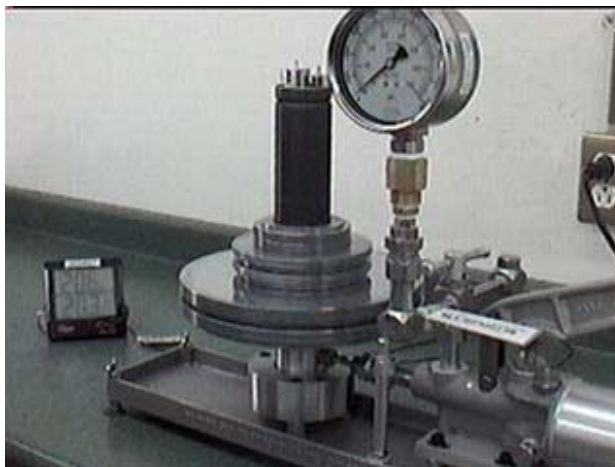
Balanza de Presión (Pesos Muertos)
