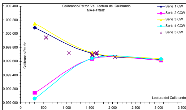
Figura 4 efecto del sentido de rotación del pistón
