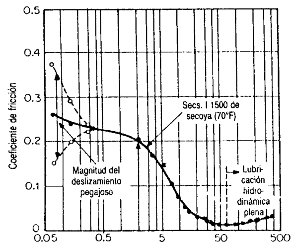
Figura 3 coeficiente de fricción Vs. frecuencia de rotación en \text{min}^{-1} [10]
