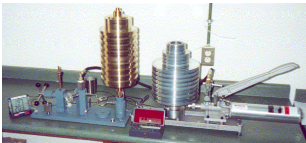
Figura 2 calibración por flotación cruzada
